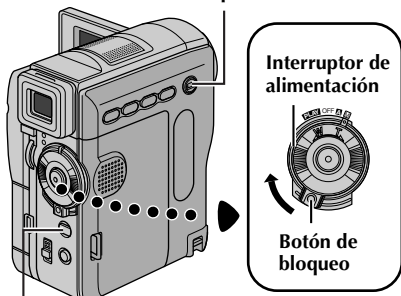
Botón SNAPSHOT
