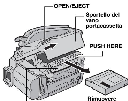
Vano portacassetta
