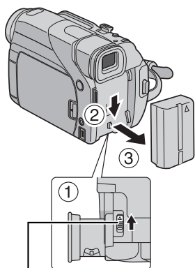
BATT.RELEASE
