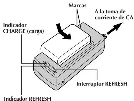
Indicador REFRESH
